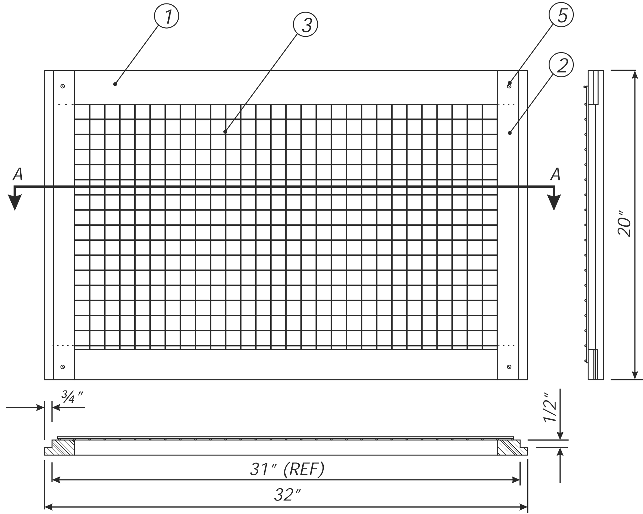
SECTION A-A
